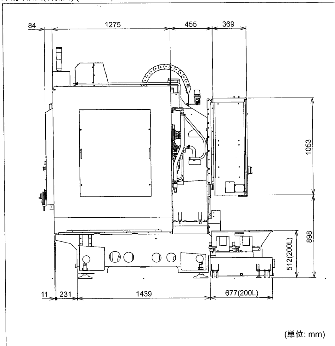
外觀寸法図(右側面) (S1000X1)
