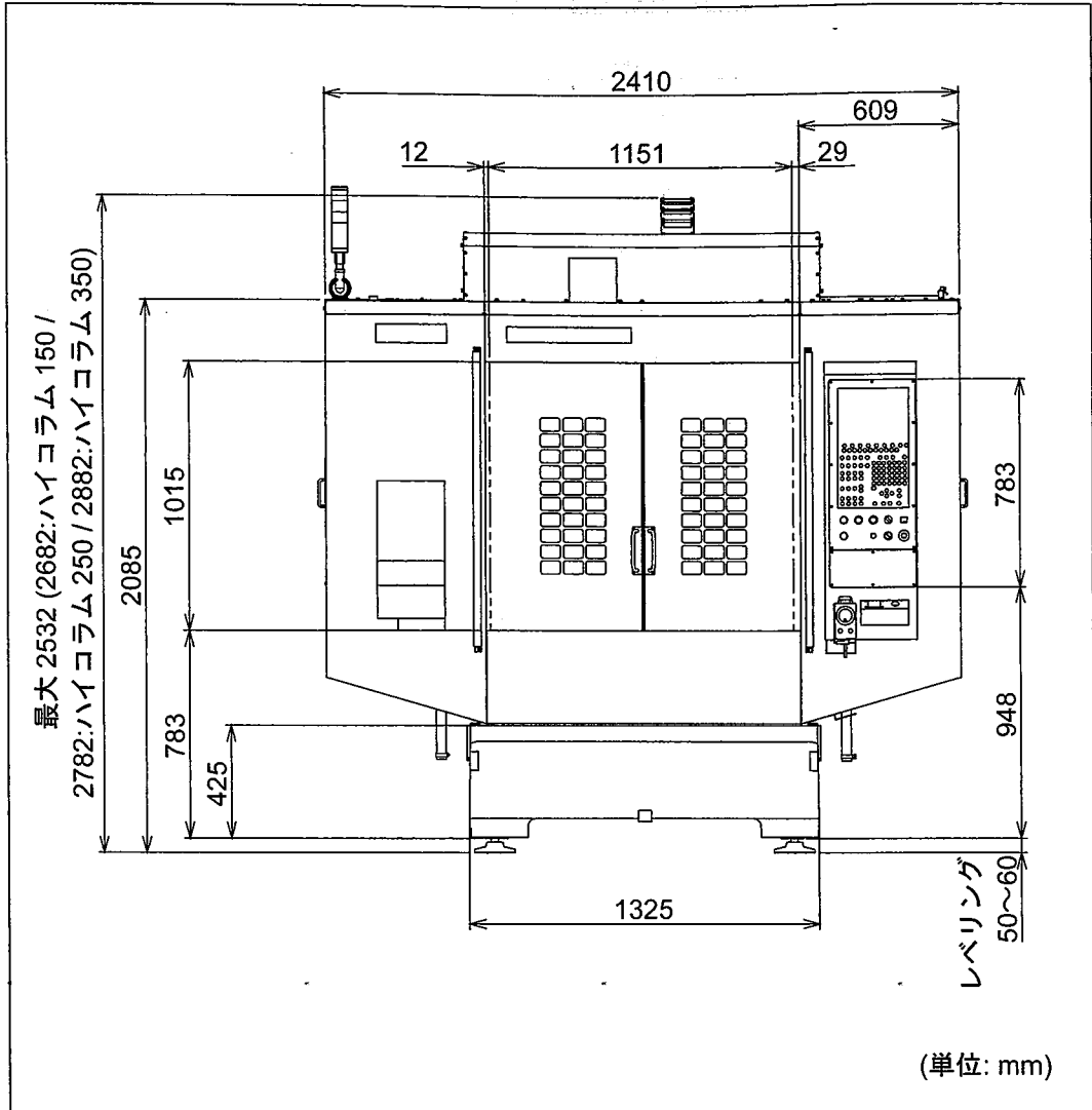
主要寸法(正面) (S1000X1)
