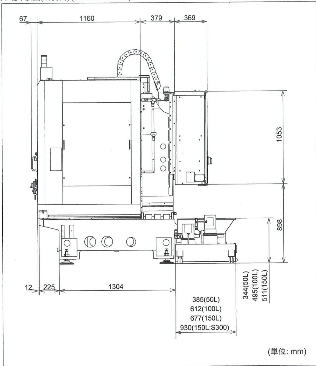
外觀寸法図(右側面) (S300/500/700X1)
