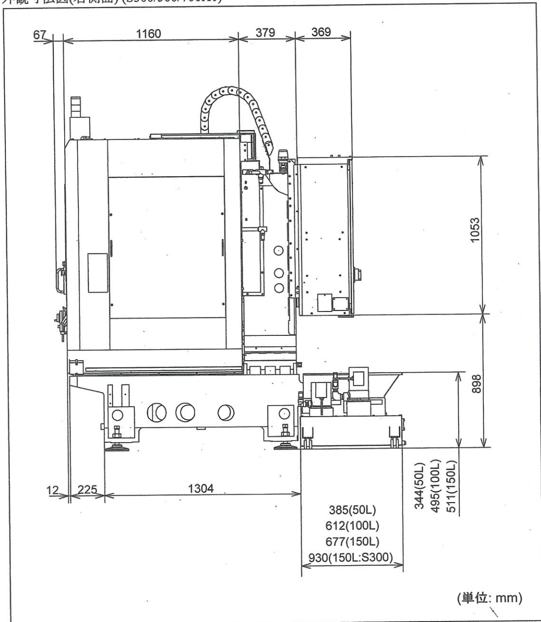
外觀寸法図(右側面) (S300/500/700X1)
